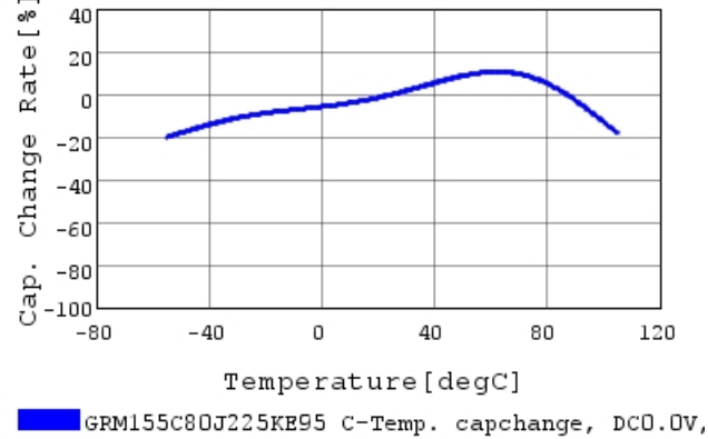
温度特性
